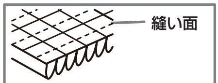
エアフィルター (細目)
