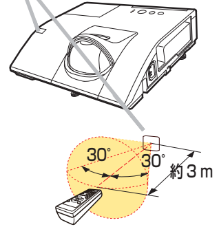
リモコン受光部
