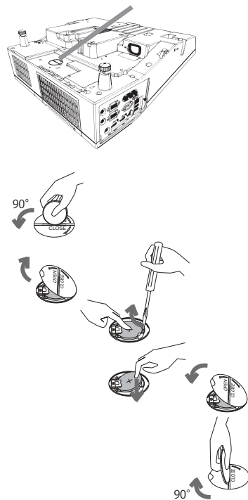
電池カバー
