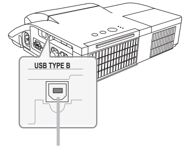
USB TYPE B 端子
