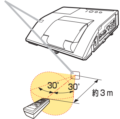
リモコン受光部
