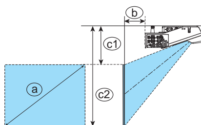
天吊り (天井設置)、または壁掛けで
